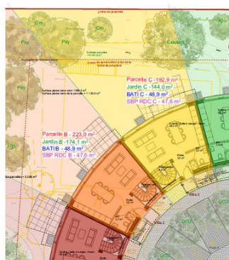
Rez-de-chaussée
